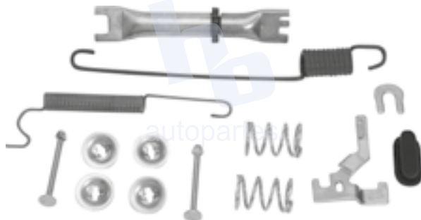
KIT PARA FRENO DE TAMBOR RUEDA TRASERA CHEVROLET EQUINOX (05-07) 1500 S780.
