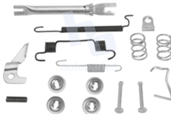
KIT PARA FRENO DE TAMBOR RUEDA TRASERA CHEVROLET AVEO (04-17), OPTRA (04-06), SONIC (12-13), SPARK (10-18) 1547 S814.
