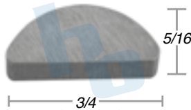
autopartes CUÑA PARA CIGÜEÑAL DE MEDIA LUNA PARA CHEVROLET C15 (82-88)
