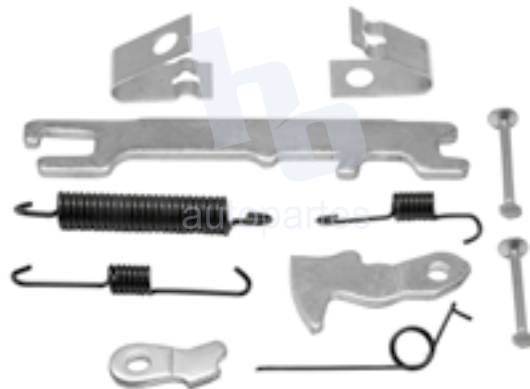
KIT PARA FRENO DE TAMBOR RUEDA TRASERA TOYOTA ECHO (01-05) BX754 S754.
