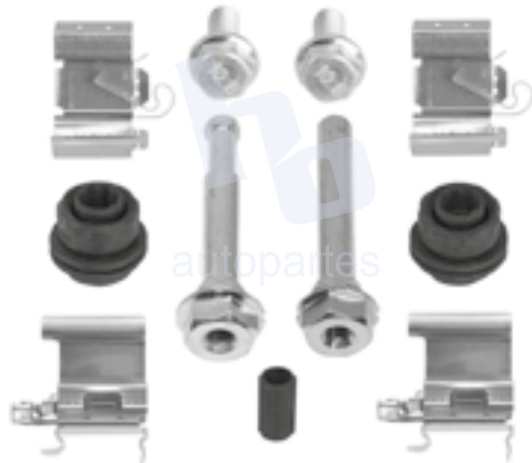
KIT DE CALIPER RUEDA TRASERA FIAT 500X, JEEP RENEGADE (15-16) 9044 D1809.
