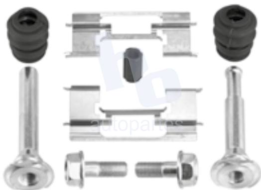
KIT DE CALIPER RUEDA DELANTERA CHRYSLER PACIFICA (04-07) 7898 D997.
