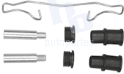
KIT DE CALIPER RUEDA DELANTERA RENAULT CAPTURE 2.0L (18-20), DUSTER (13-16), FLUENCE (11-13), OROCH (19-20) 8844 D1627.
