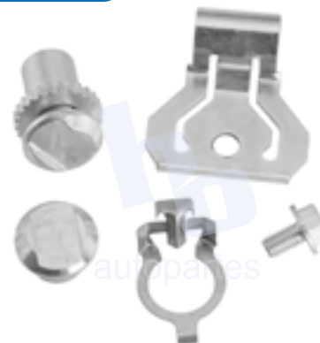
KIT PARA FRENO DE ESTACIONAMIENTO RUEDA TRASERA CADILLAC ESCALADE (04-07), CHEVROLET AVALANCHE (07-13), GMC SIERRA 1500 (07-10), YUKON XL 2500 (07-10), YUKON 4WD (07-10) 2196 781.
