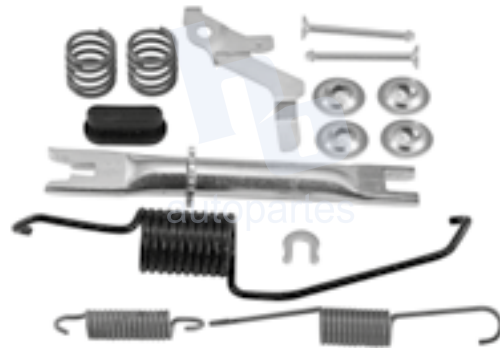
KIT PARA FRENO DE TAMBOR RUEDA TRASERA TOYOTA COROLLA (14-19), PRIUS C (14-18) 1635 S945.
