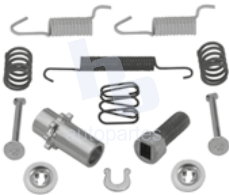
KIT PARA FRENO DE ESTACIONAMIENTO RUEDA TRASERA MITSUBISHI OUTLANDER (07-12) 1601 887.
