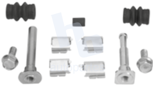
KIT DE CALIPER RUEDA DELANTERA CHRYSLER GRAND VOYAGER (01-06), DODGE CARAVAN RIN 15 (01-06), 7732 D856. KIT DE CALIPER RUEDA TRASERA JEEP LIBERTY (02-06) 7732 D856.
