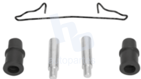
KIT DE CALIPER RUEDA DELANTERA KIA SEPHIA (94-01) 7529 D649.
