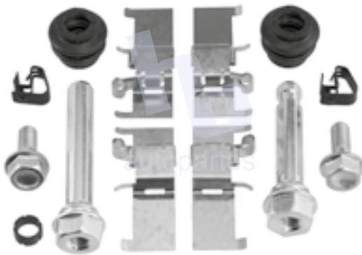
KIT DE CALIPER RUEDA DELANTERA LEXUS ES 300H (13-18) 8331 D1293, TOYOTA AVALON (15-16) 8331 D1222, CAMRY (07-17) 8331 D1293.
