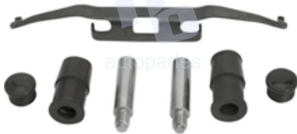
KIT DE CALIPER RUEDA DELANTERA MERCEDES BENZ SPRINTER (04-06) 7849 D950.
