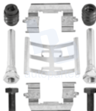
KIT DE CALIPER RUEDA DELANTERA ACURA CL (01-03), HONDA ACCORD EX 6 CIL (03-09) 7556 D787, ACCORD HYBRID (06-07) 7656 D787.
