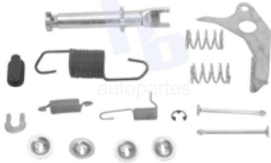
KIT PARA FRENO DE TAMBOR RUEDA TRASERA MITSUBISHI MONTERO (89-95), PICK UP (87-95) 1370 524.
