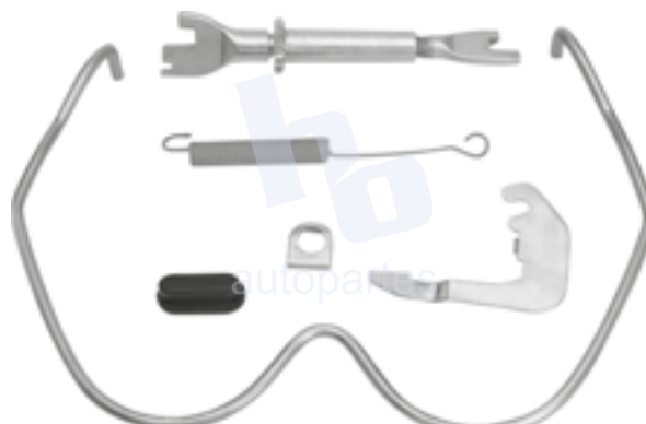
KIT PARA FRENO DE TAMBOR RUEDA TRASERA CHEVROLET COLORADO (04-08) 1548 S855, SILVERADO 1500 (05-08), GMC SIERRA 1500 (05-08), ISUZU DMAX 2WD (04-07) 1548 S815.
