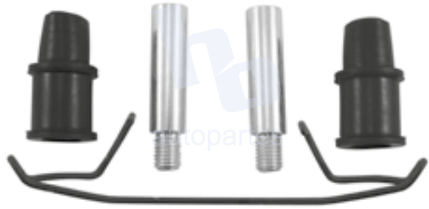
KIT DE CALIPER RUEDA DELANTERA FORD ESCAPE (01-06), FORD MARINER (06-07) 7719 D843.
