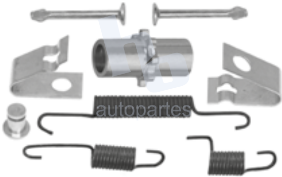
KIT PARA FRENO DE TAMBOR RUEDA TRASERA HONDA CR-V (07-16) 1588 S928.
