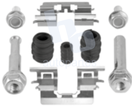
KIT DE CALIPER RUEDA DELANTERA SUBARU FORESTER 2.0L (14-16), SUBARU LEGACY (14-15) 7983 D1078.
