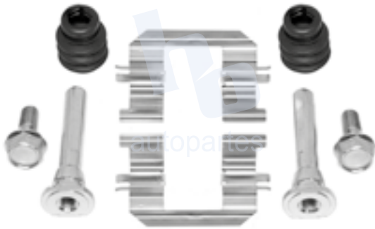
KIT PARA CALIPER RUEDA DELANTERA CHEVROLET SPARK NG (16-20) 9083 D1684, 9254 D2024.
