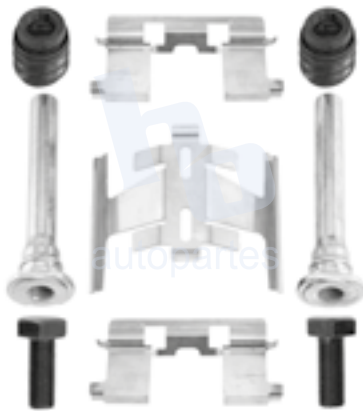
KIT DE CALIPER RUEDA DELANTERA HONDA ACCORD (91-02), ODYSSEY (95-98) 7382 D503.
