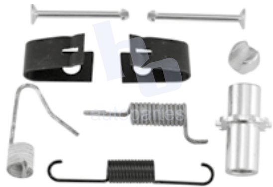
KIT PARA FRENO DE TAMBOR RUEDA TRASERA TOYOTA AVALON (13-16), CAMRY (12-17) 1691 S1024.
