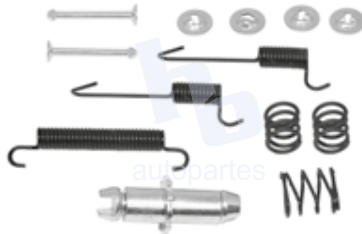
KIT PARA FRENO DE ESTACIONAMIENTO RUEDA TRASERA HYUNDAI TUCSON AWD (10-15), KIA SPORTAGE (11-16) 1662 S988.
