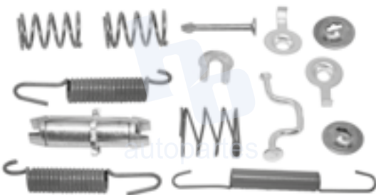
KIT PARA FRENO DE ESTACIONAMIENTO RUEDA TRASERA TOYOTA 4RUNNER (05-16), FJ CRUISER (06-14), SEQUOIA (08-14) 1580 S850.
