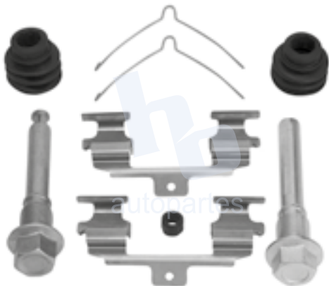
KIT DE CALIPER RUEDA DELANTERA NISSAN QUEST (04-17) 7910 D855, 8762 D1552.
