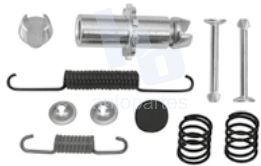
KIT PARA FRENO DE TAMBOR RUEDA TRASERA CADILLAC ESCALADE (15-20), CHEVROLET SIERRA 1500 (13-18), SILVERADO 1500 (13-18), SUBURBAN (15-17) TAHOE (15-17), GMC SIERRA (17-18), SILVERADO 1500 (13-18), YUKON (15-20), YUKON XL (15-17) 1710 S1051.
