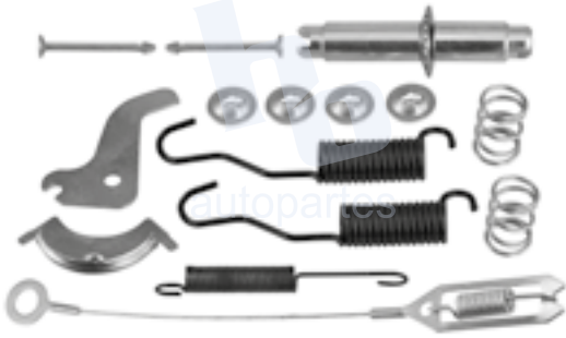
KIT PARA FRENO DE TAMBOR RUEDA TRASERA TOYOTA PICKUP (79-83) 2156 523.
