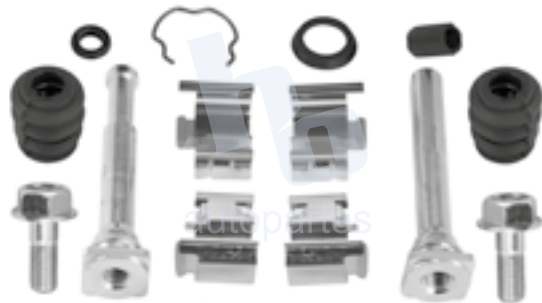
KIT DE CALIPER RUEDA TRASERA TRANSIT (15-18), TRANSIT 150 (15-18), TRANSIT 250 (15-18), TRANSIT 350 (15-18), TRANSIT 350 HD (15-18) 9005 D1775
