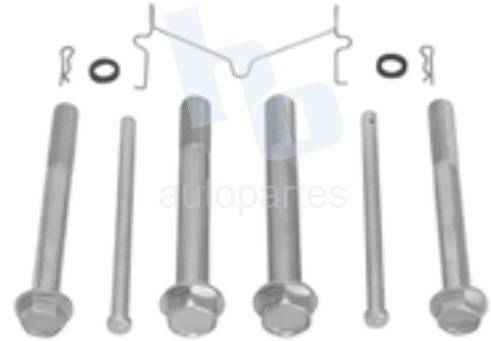
KIT DE CALIPER RUEDA DELANTERA AM GENERAL HUMMER H2 (06-09), HUMMER H3 (06-10), HUMMER H3T (06-12) 8225 D1119.
