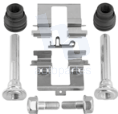
KIT DE CALIPER RUEDA DELANTERA ACURA MDX V6 3.7L (14-16), ACURA ZDX (10-13) 8397 D1281. KIT DE CALIPER RUEDA TRASERA HONDA ODYSSEY (11-17) 8397 D1281.
