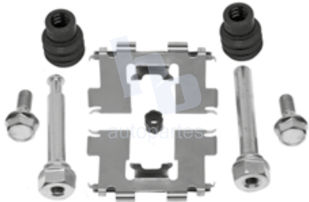
KIT DE CALIPER RUEDA DELANTERA CHEVROLET CRUZE (16-18), VOLT (16-17) 9072 D1844.
