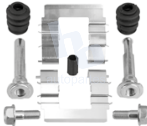
KIT DE CALIPER RUEDA DELANTERA DODGE ATTITUDE (06-07), HYUNDAI ACCENT (06-09), KIA RIO (06-09) 8266 D1156.
