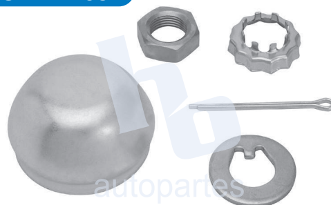
KIT DE SEGUROS Y TUERCA (1) RUEDA DELANTERA CHEVROLET LUV (00-05), ISUZU AMIGO (89-94), TROOPER (89-91), RODEO (91-95), HONDA PASSPORT (94-95)
